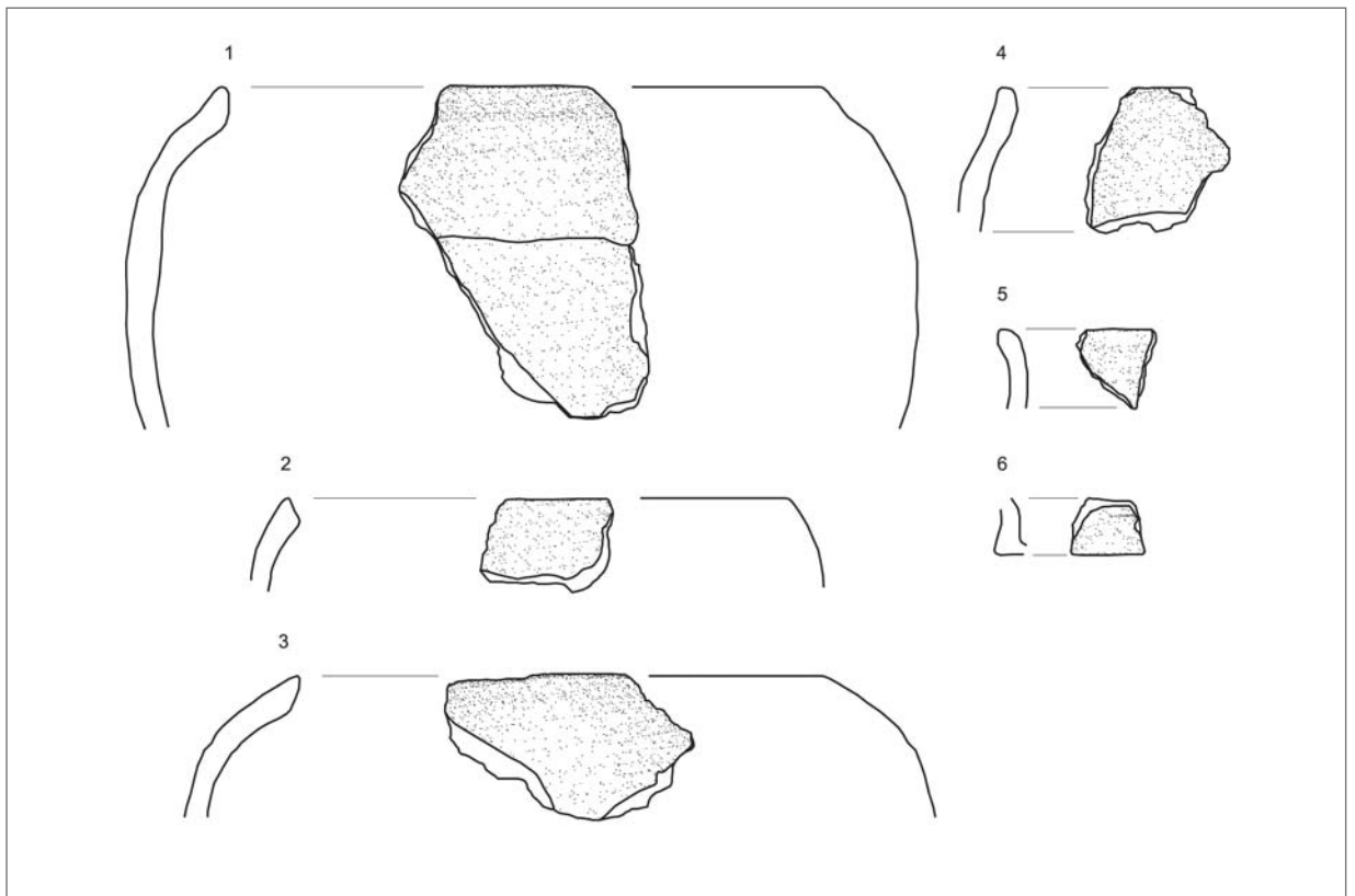
Abb. 3: Paderborn, Spitalmauer 10, Keramikscherben, M. 1:3.
