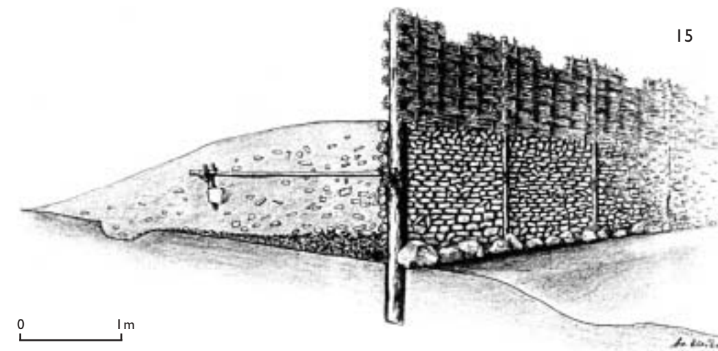
Abb. 9 Rekonstruktion einer Burgmauer aus der vorrömischen Eisenzeit nach Befunden der Hünenburg bei Bielefeld.
